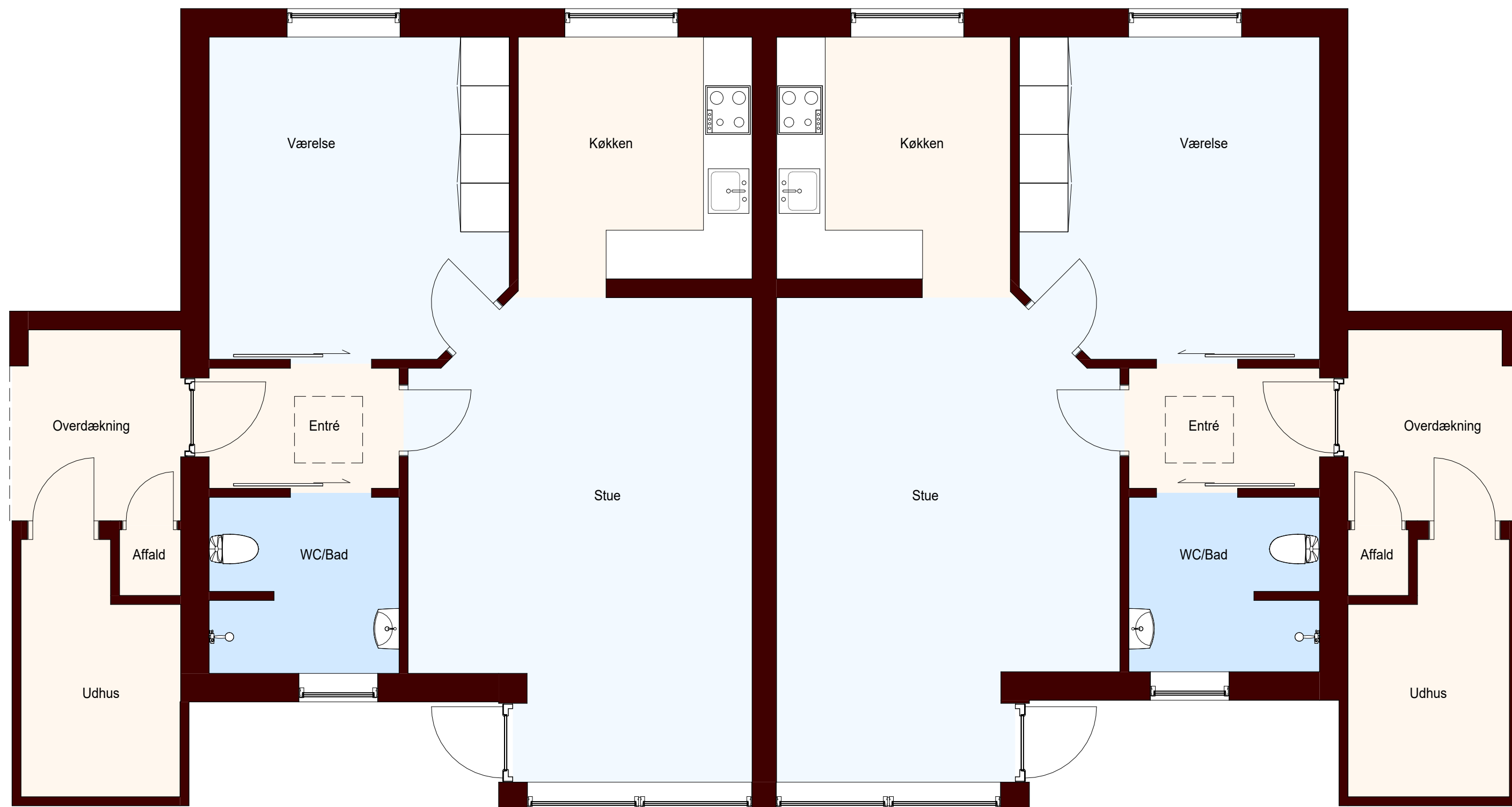
Stueplan - Dobbelthus 1:50
