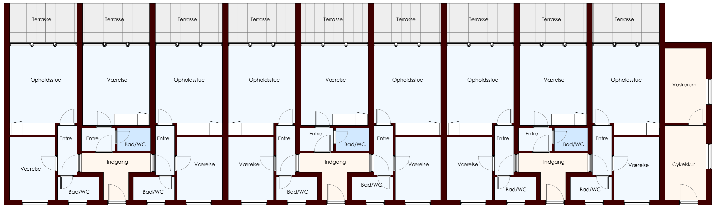
Stueplan 1:100
