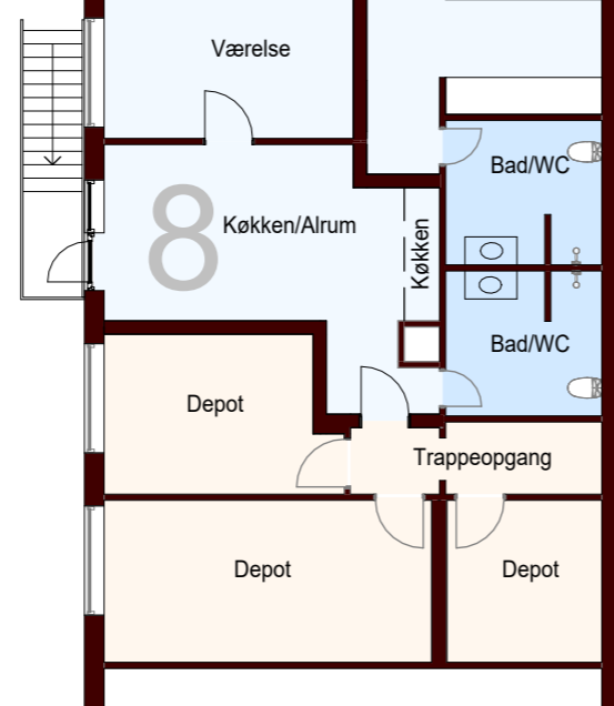
LEJLIGHEDSFLØJ 1. SAL 1:150
