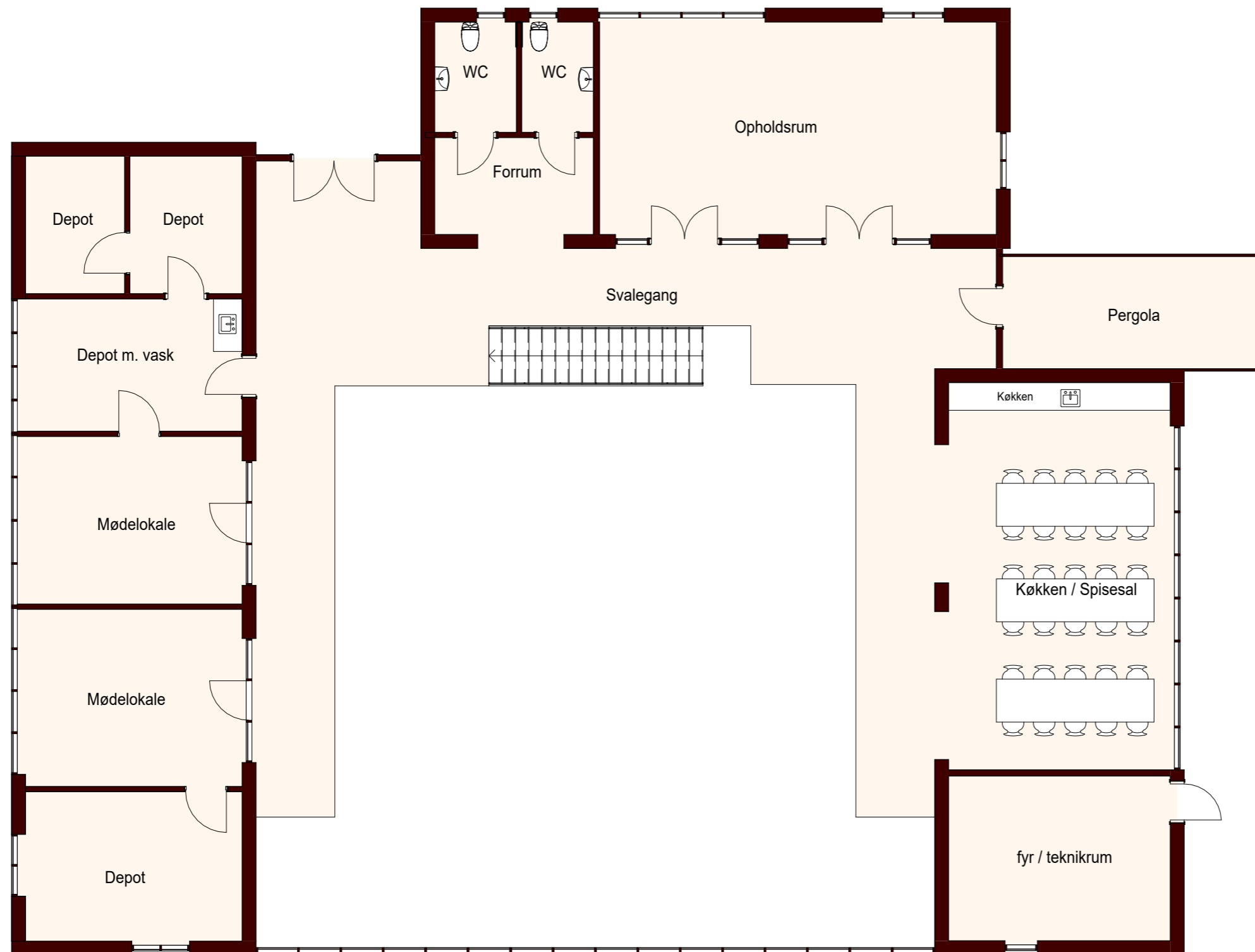
1. Sal - Aktivitetshus 1:150
