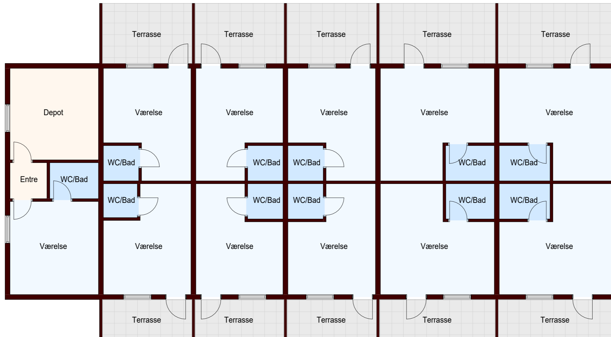
Stueplan 1:100
