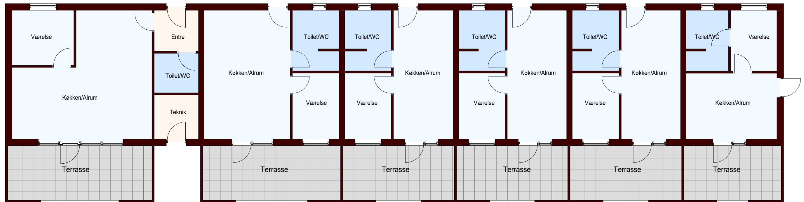
Beboelsesfløj Syd Stueplan 1:100
