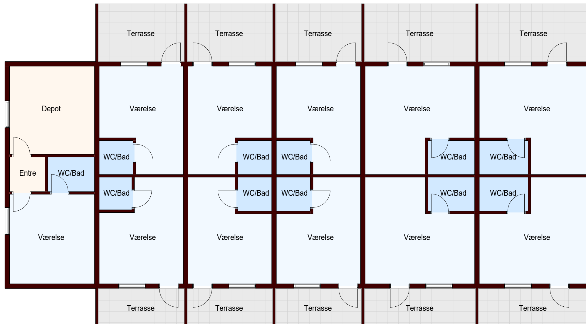
Stueplan 1:100
